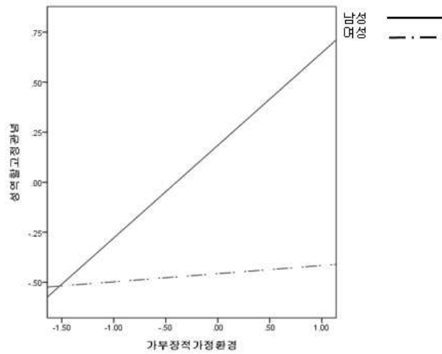
그림 1. 가부장적 가정환경과 성역할 고정관념 관계에서 성별의 조절효과
