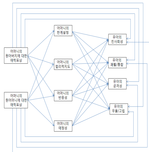
그림 1. 연구 가설모형
