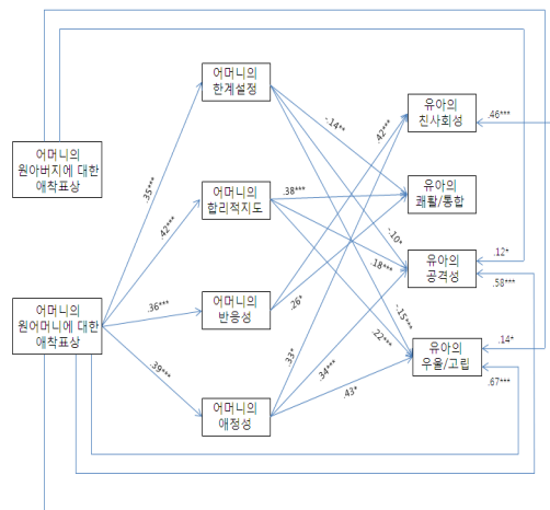
그림 2. 연구 수정모형
